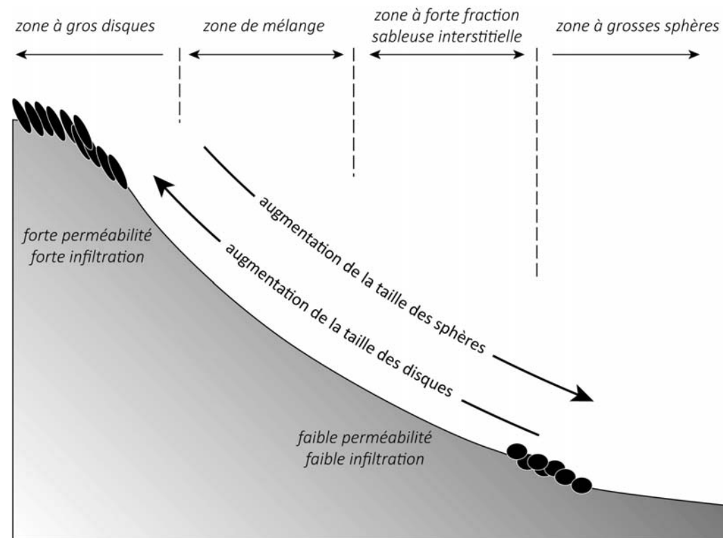
Figure 4 : Profil type d'un cordon de galets où sont résumées les caractéristiques du tri des galets selon leur forme et leur taille telles que l'envisage Bluck (1967) (modifié de Bluck, 1999).
